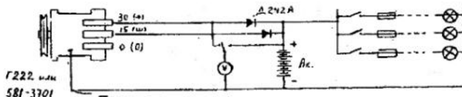
Подключение генератора со встроенным регулятором напряжения.
